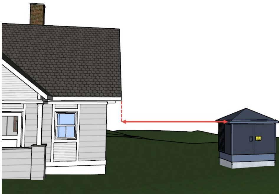
Figur 5 Det er krav til minimum 5 meter avstand fra nettstasjon til annen bygning
